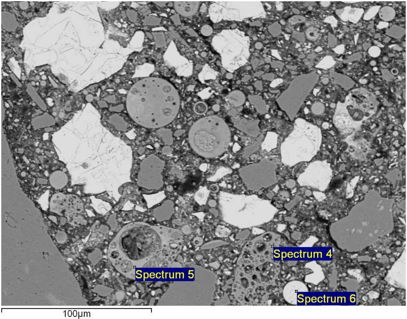
Figura 3A-eletromicrografia SEM-EDS na seção fina. Matriz compacta entre os componentes e o "efeito parede" cimento pozolânico (contatos entre as massas)-colar.
