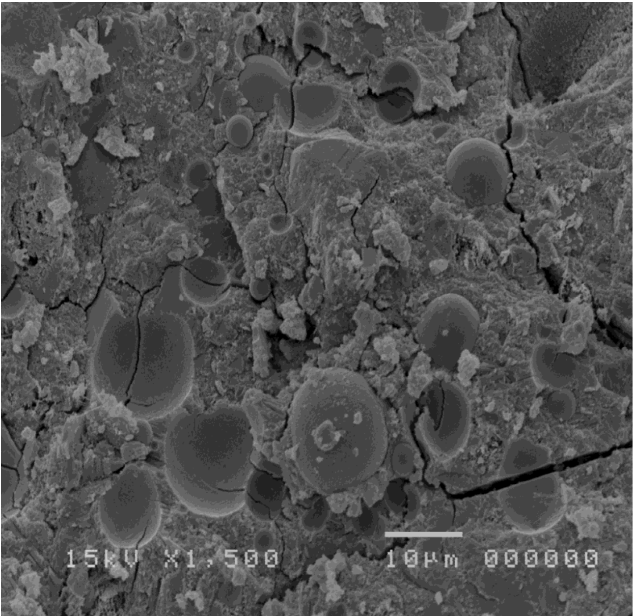
Figura 3-F-SEM Micrografia-massas-Pozzolanico pozolânico matriz muito compacto
