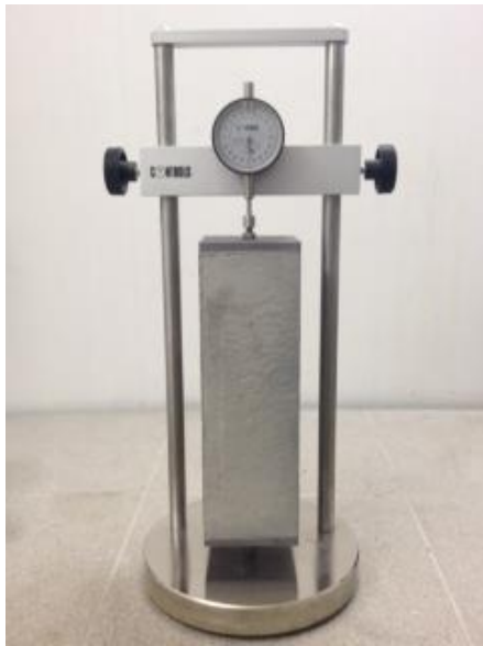
Foto X + Y – Teste expansão contrastada
