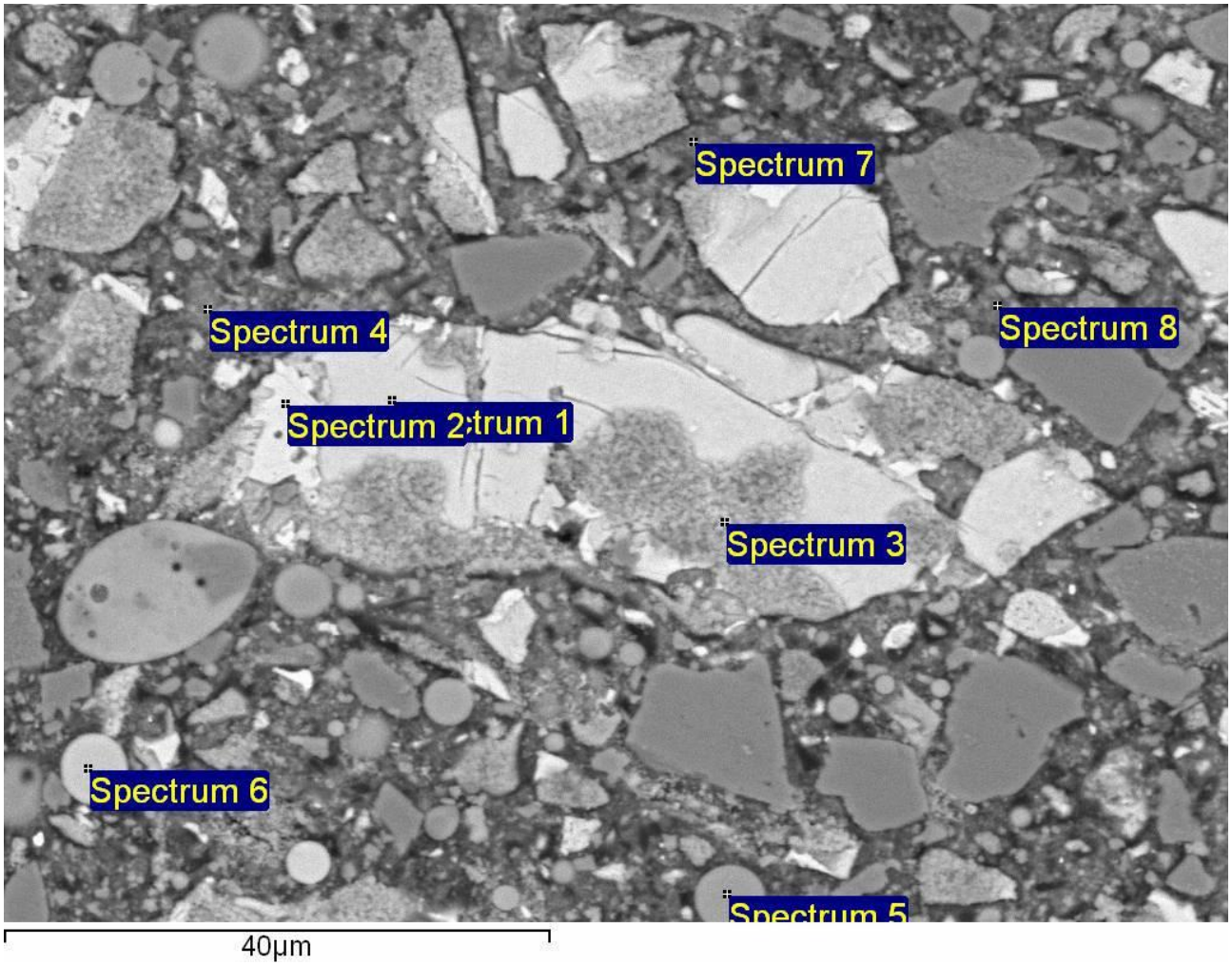
Figura 3B-eletromicrografia SEM-EDS na seção fina. Matriz compacta entre os componentes e o "efeito parede" cimento pozolânico (contatos entre as massas)-colar.
