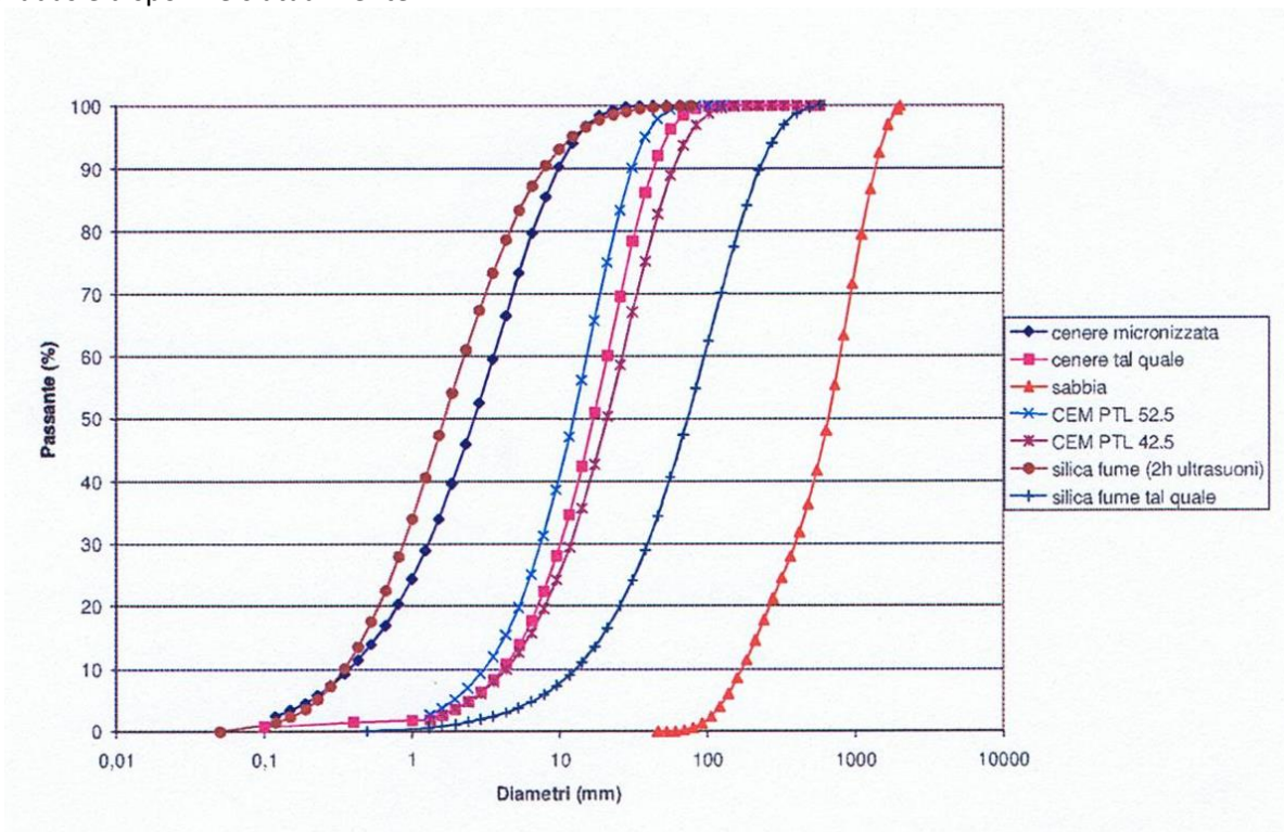
Figura: Confronto entre as distribuições granulométricas Laser de cinza nativa, cinza micronizada, cimento Portland 42.5 e 52.5, fumo de sílica (Referência e desagregado).
